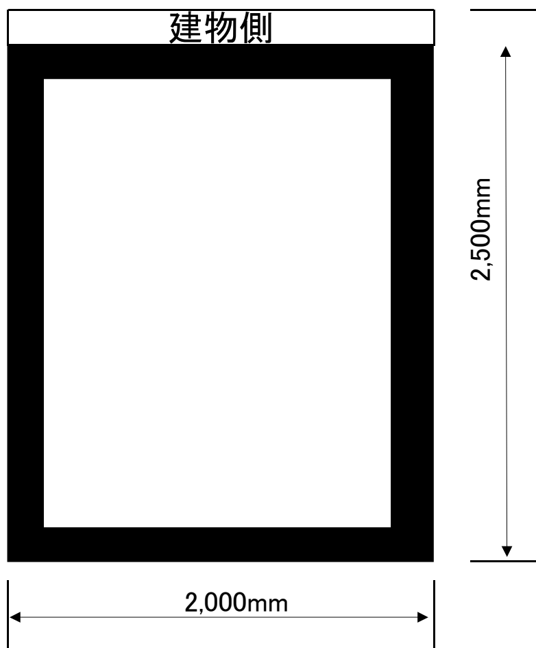
別図17 三連はしご活動空地の路面標示
