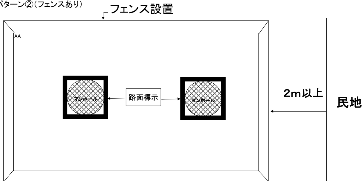
パターン②(フェンスあり)
