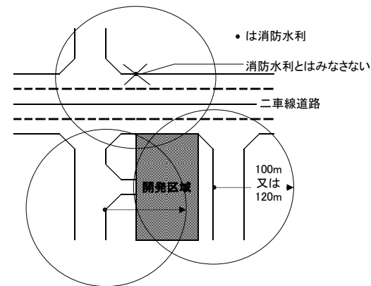
水利包含図例F(二車線道路等)
