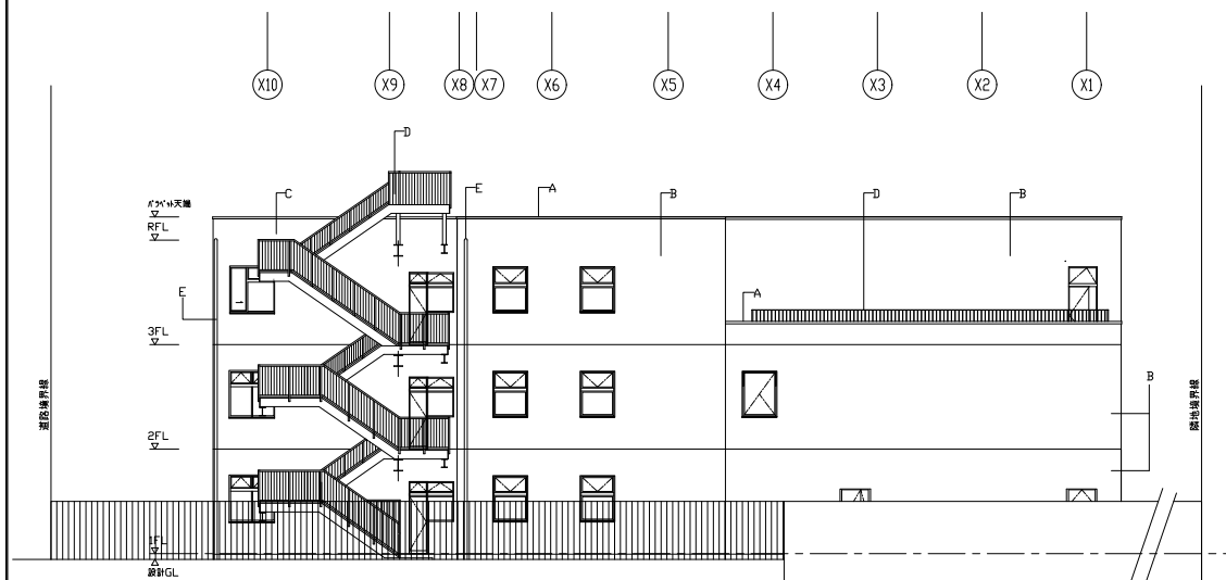
西立面図
