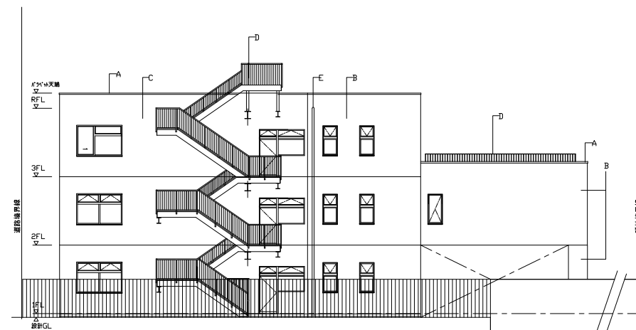
北立面図
