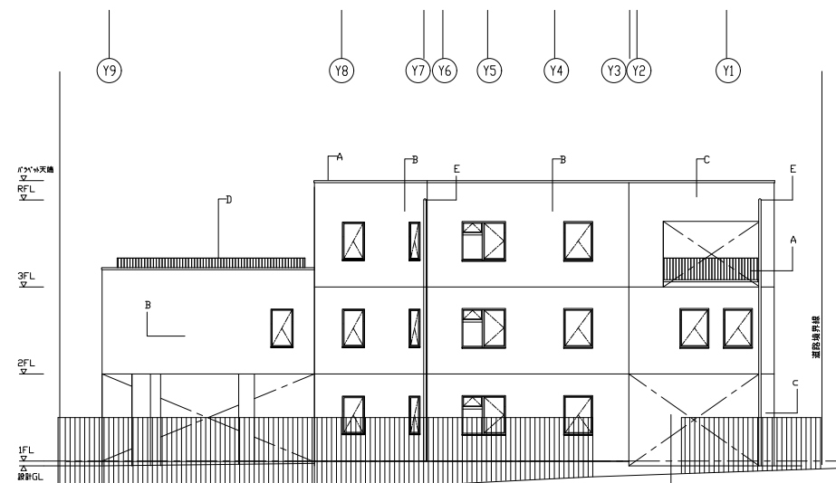
北立面図
