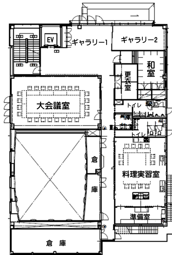
2 階
