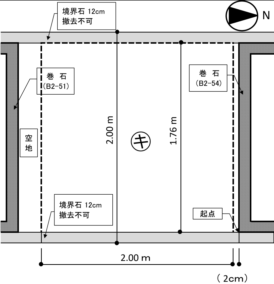
略図
