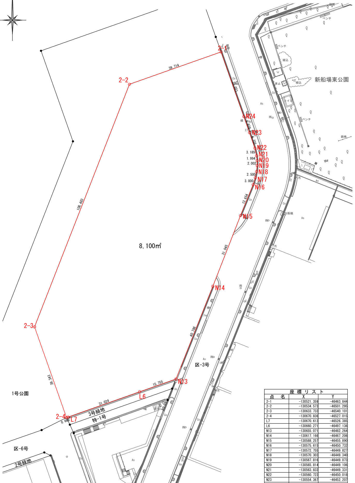
画地確定測量図 1:800
