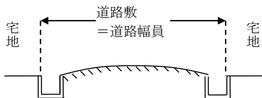
図1 U字型側溝の場合
