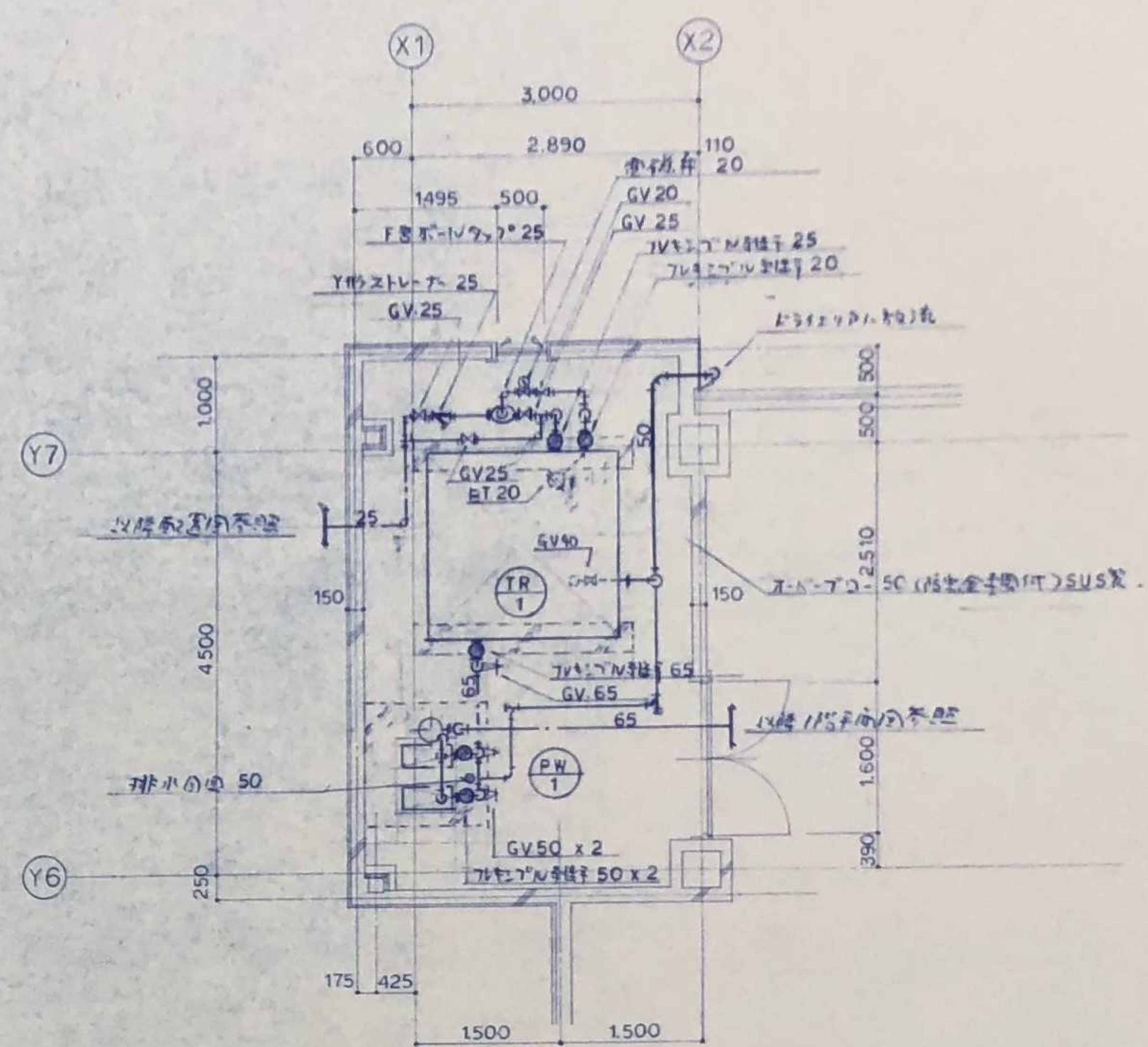
3 ポンプ室断面図
