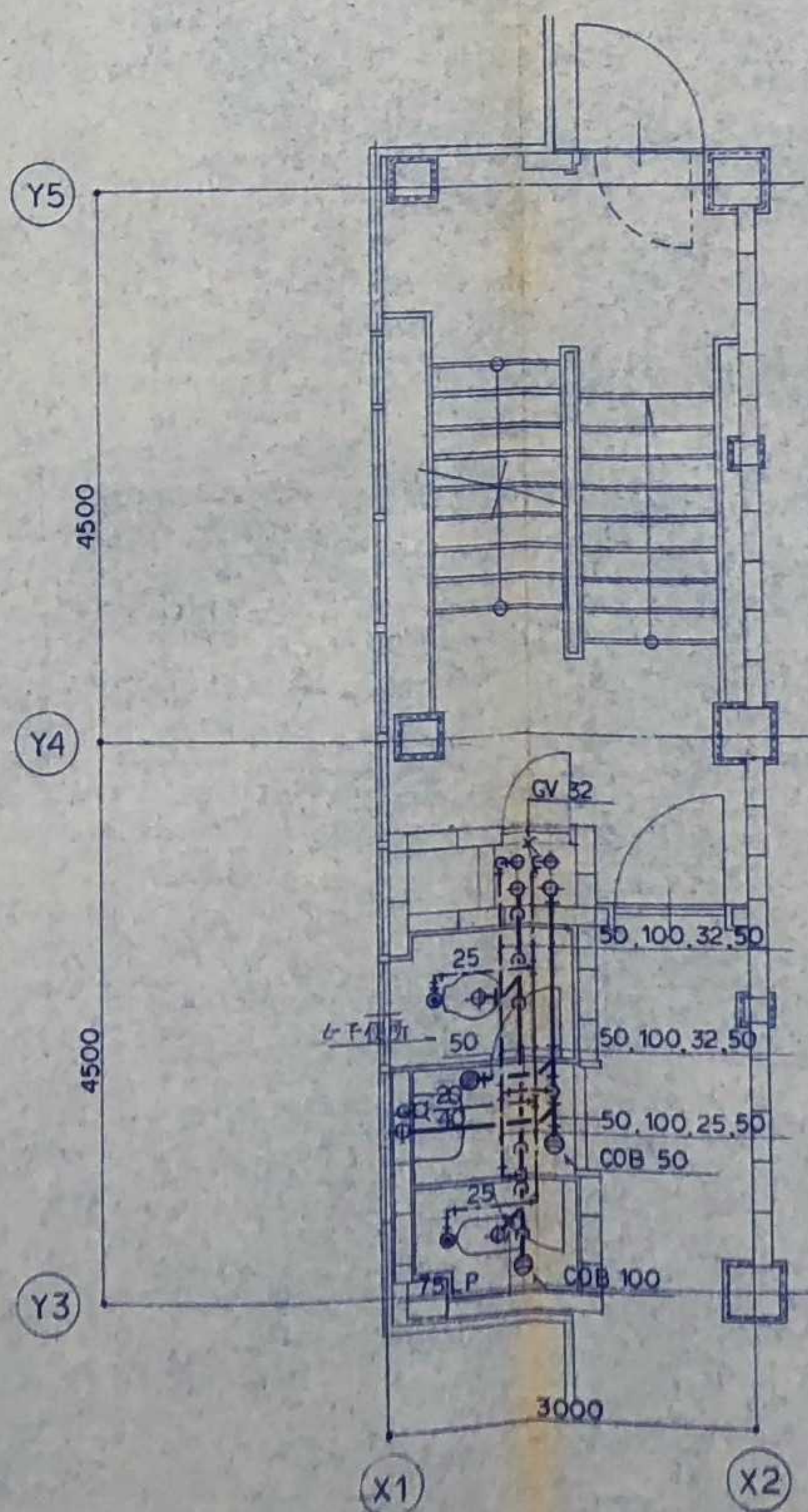
3 2~4階 女子便所 詳細図
