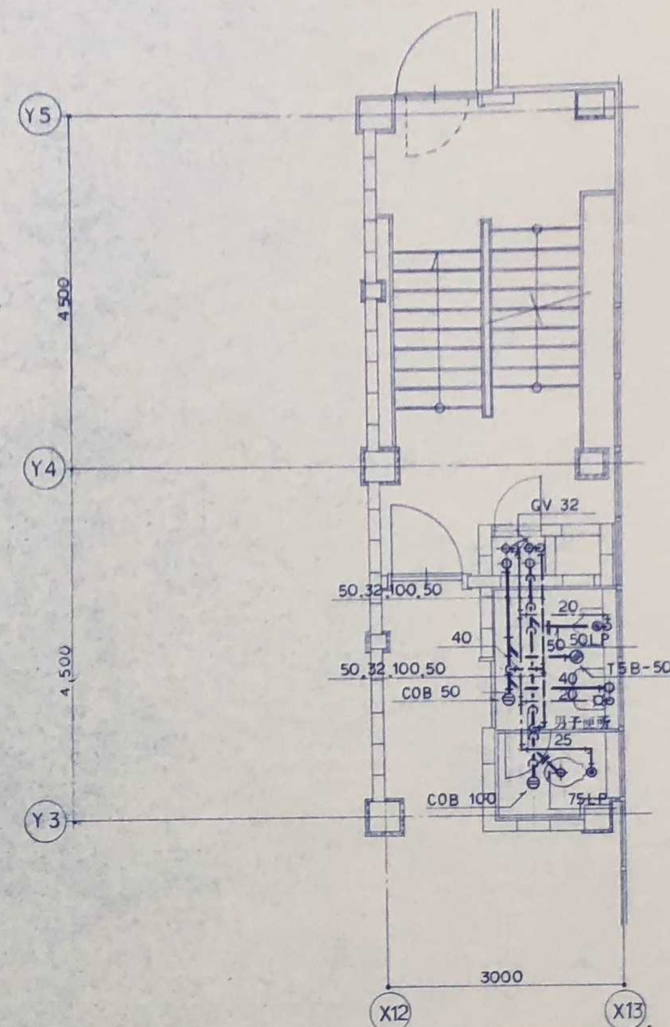
5 管理事務所 詳細図
