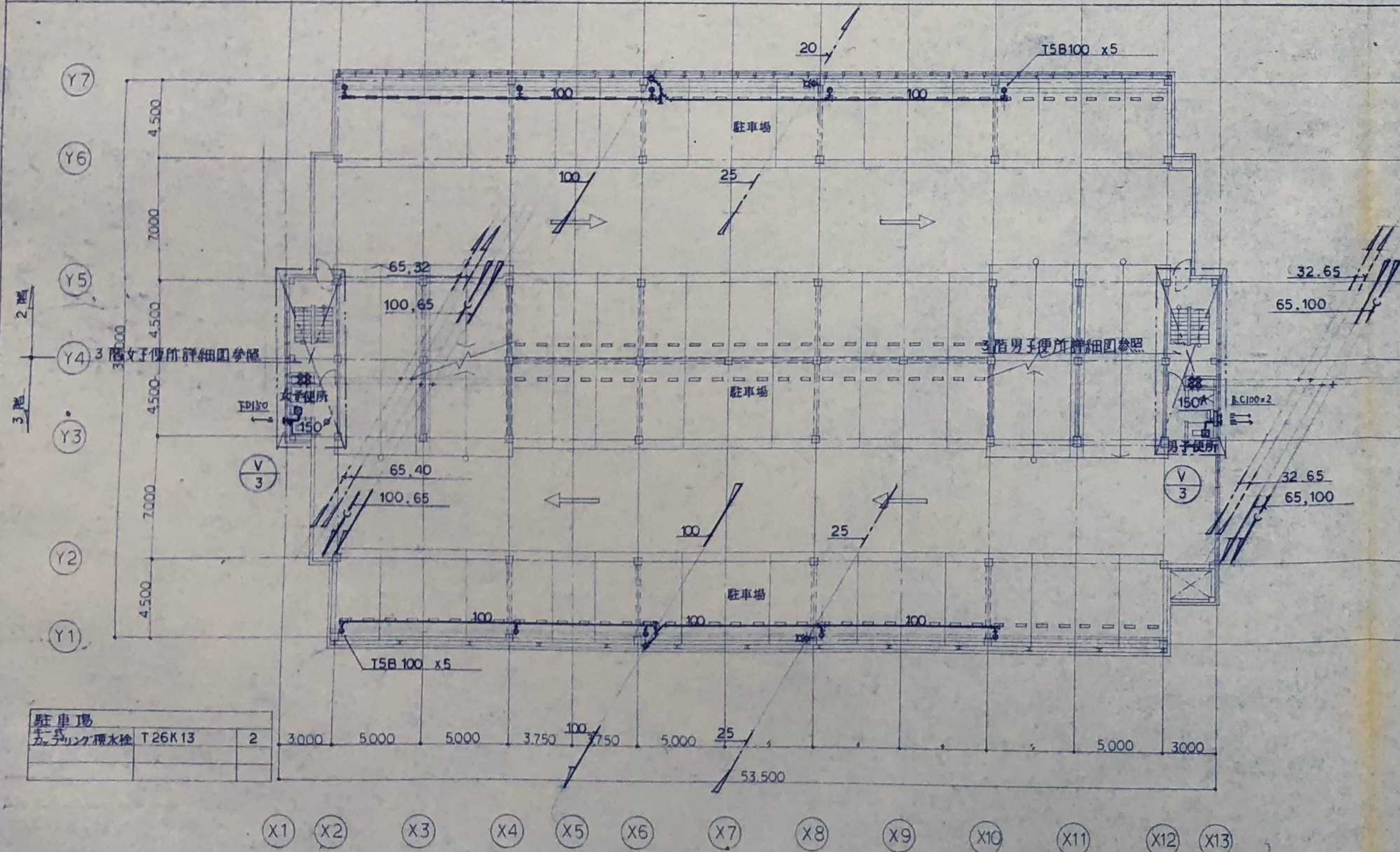
1 2,3階平面図
