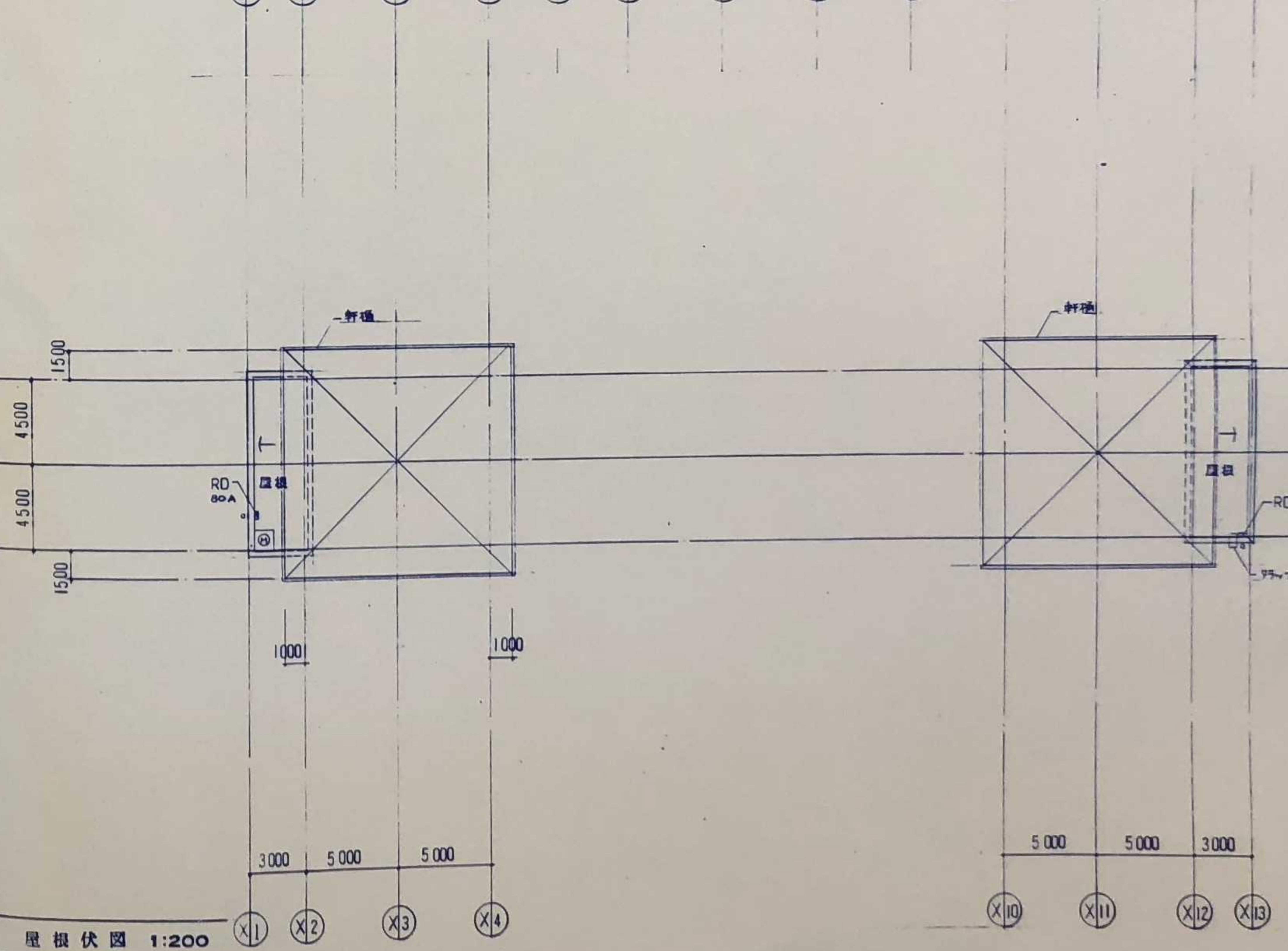
屋根伏図 1:200
