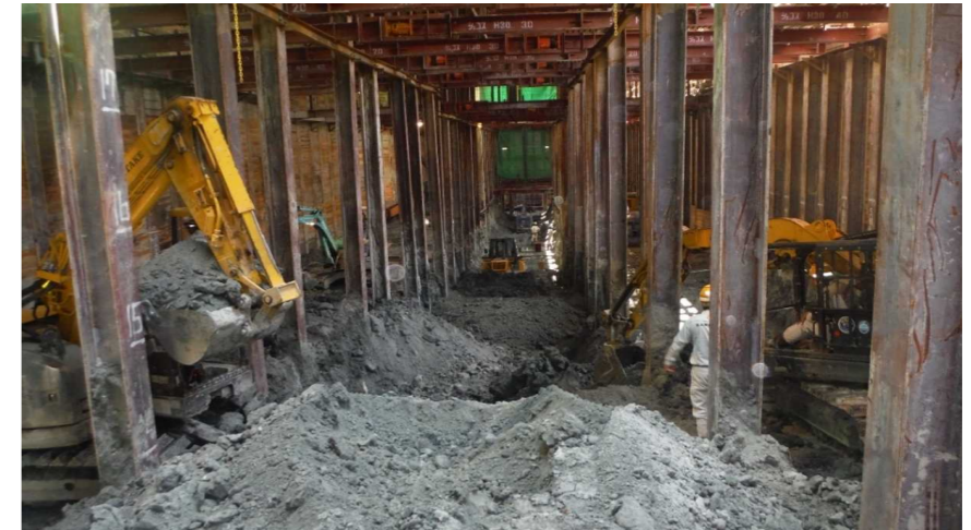
C 開削区間・箕面船場阪大前駅／視察箇所(掘削工)
