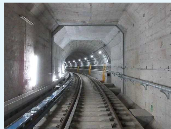
⑧トンネル区間（千里中央駅北端接続部）
