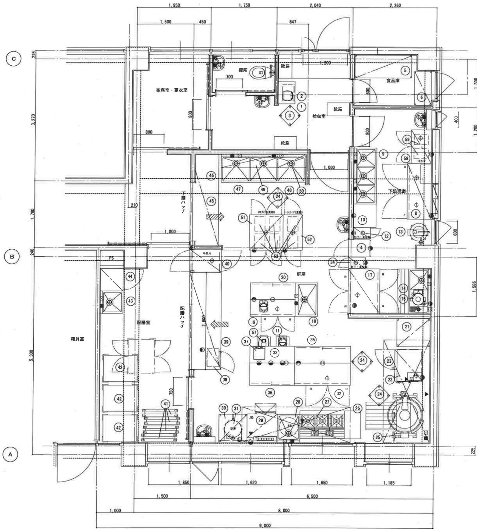
厨房機器配置図(参考図) 1/60
