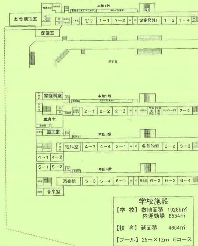
令和2年度(2020年度) 教室配置図
