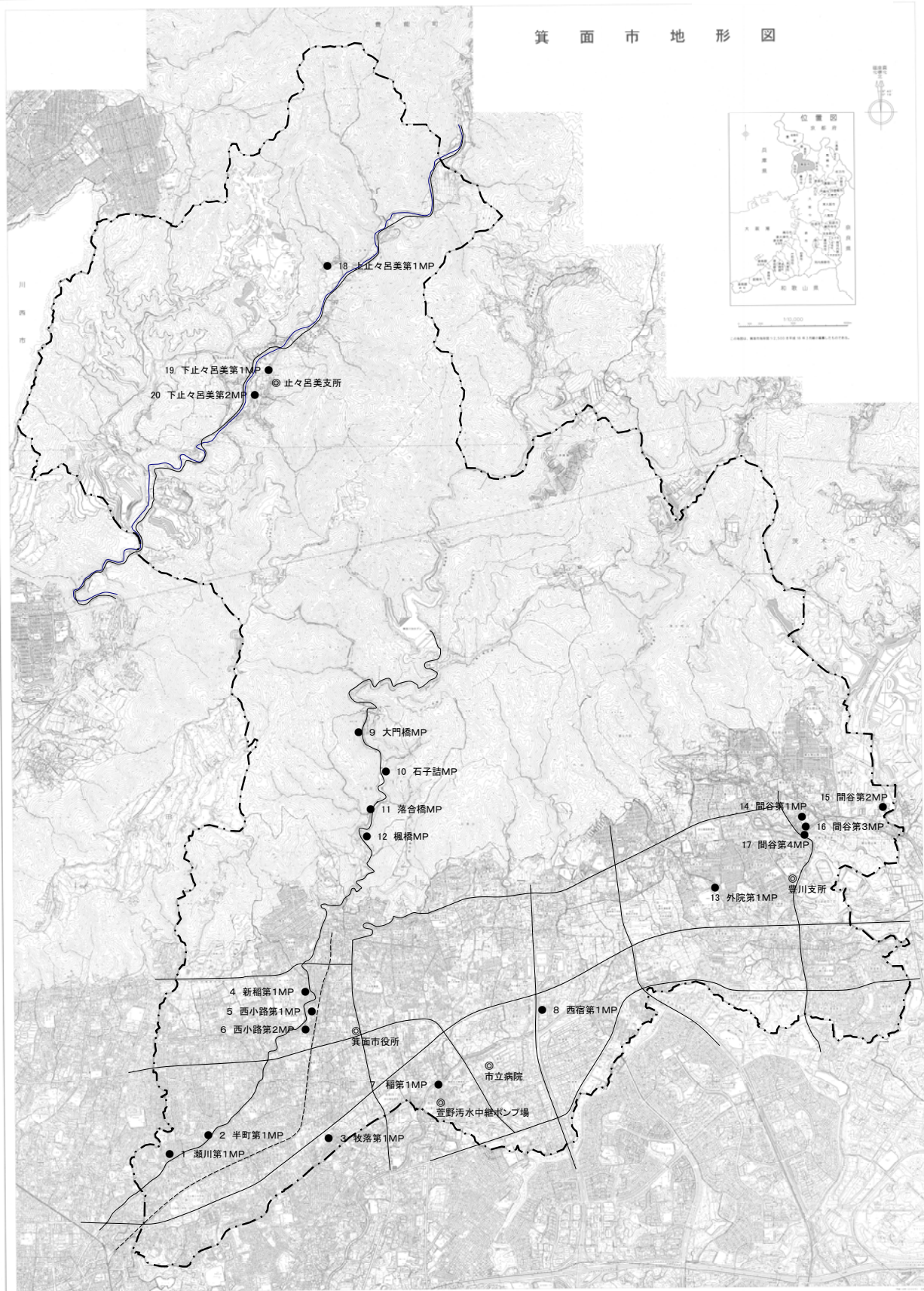
12 マンホールポンプ配置図
