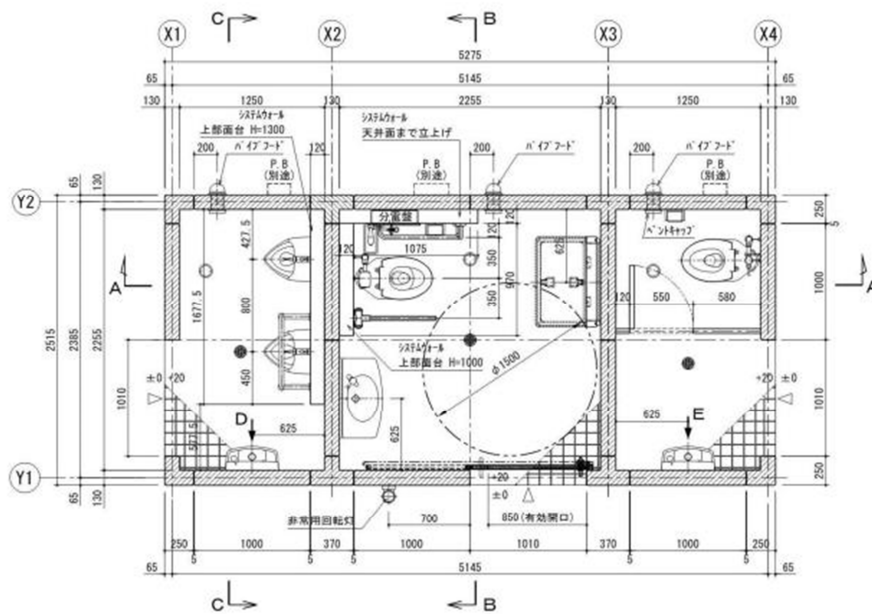
配置図（唐池公園）
