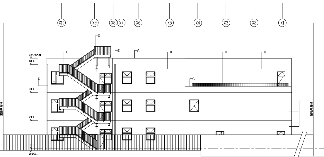
西立面図
