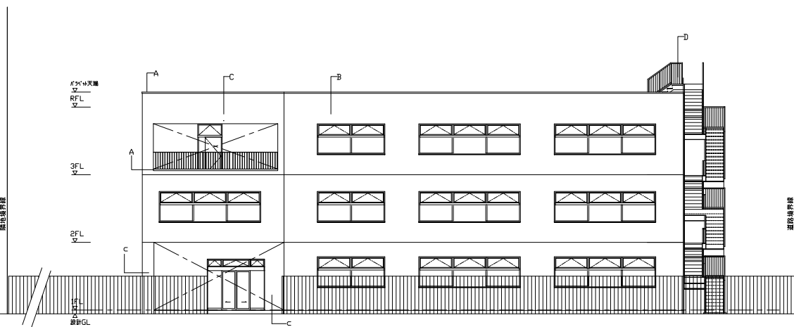
東立面図
