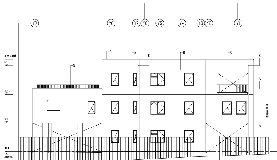
北立面図
