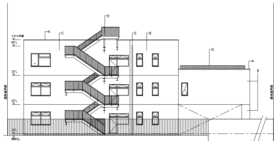
北立面図
