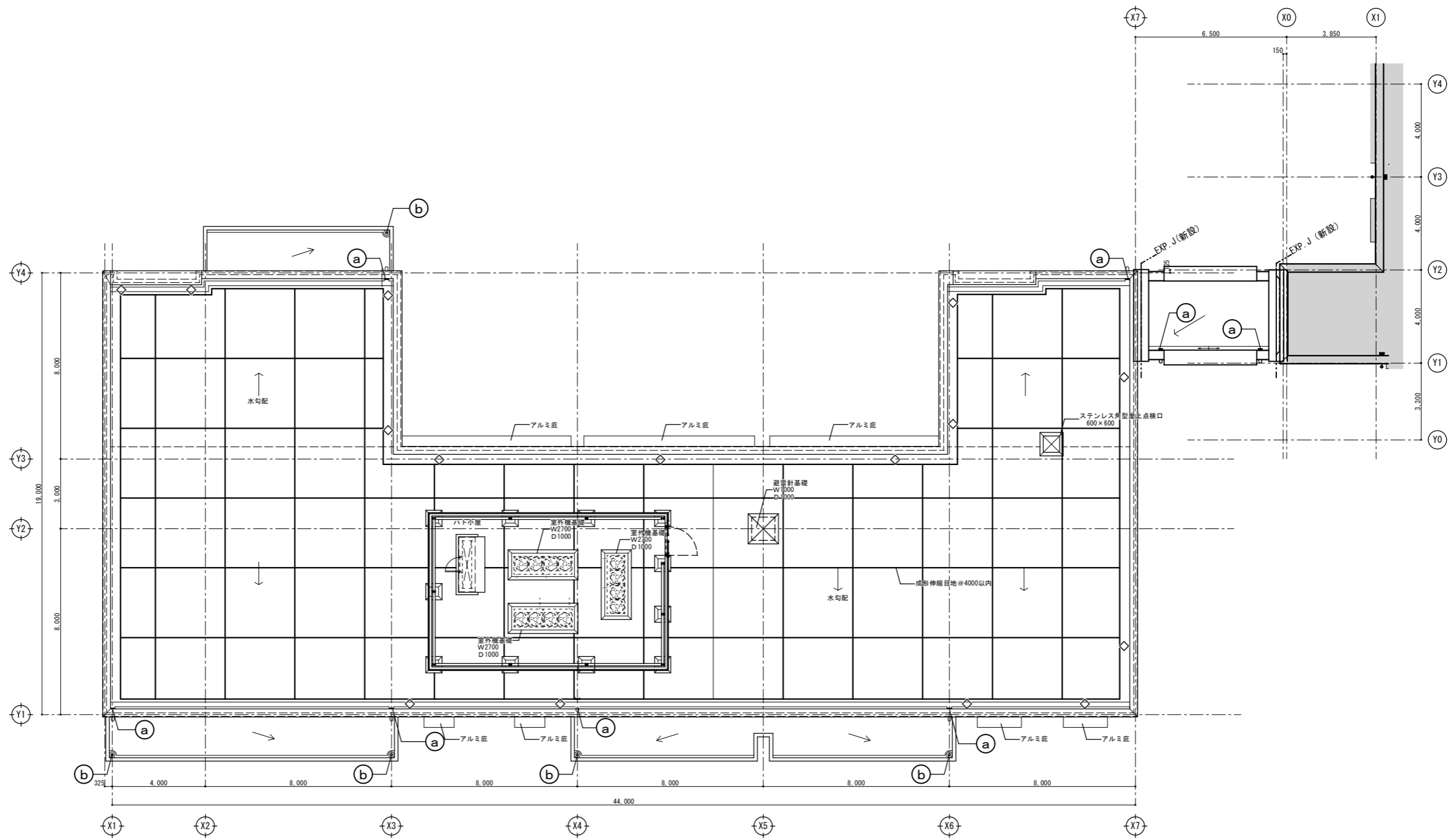
R階平面図 1/100
