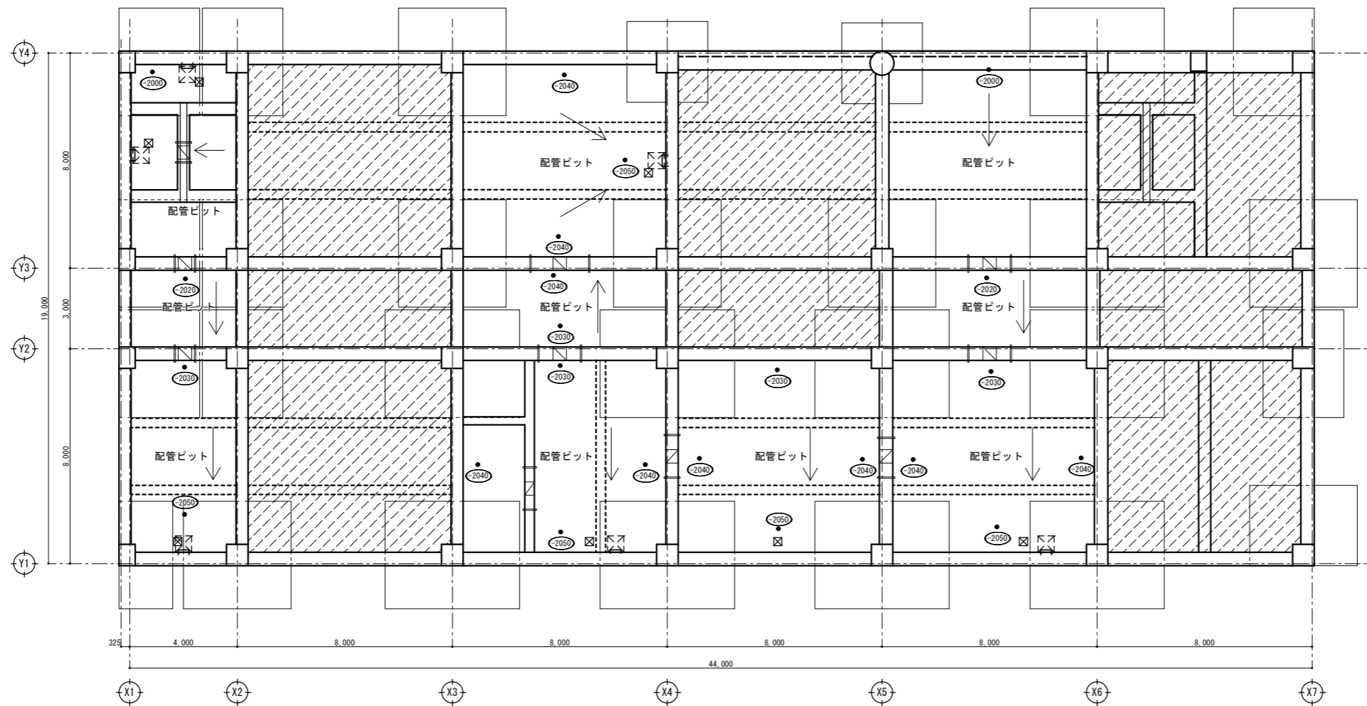
ピット平面図 1/100
